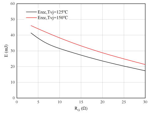
图 8. 开关损耗 二极管 Figure 8. Switching losses of Diode I_F=300A, V_{CE}=900V
